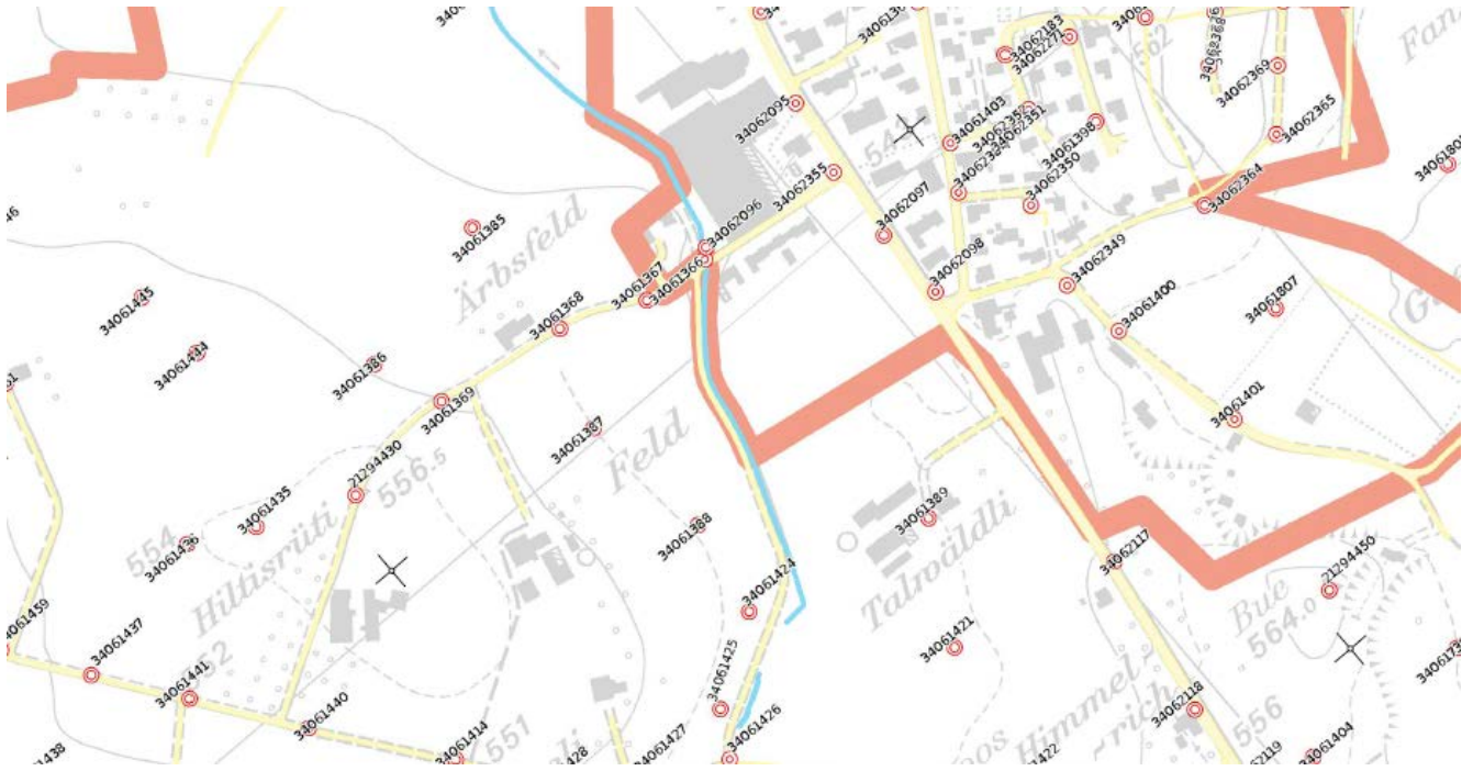
Abbildung 5: Muster Fixpunktplan
